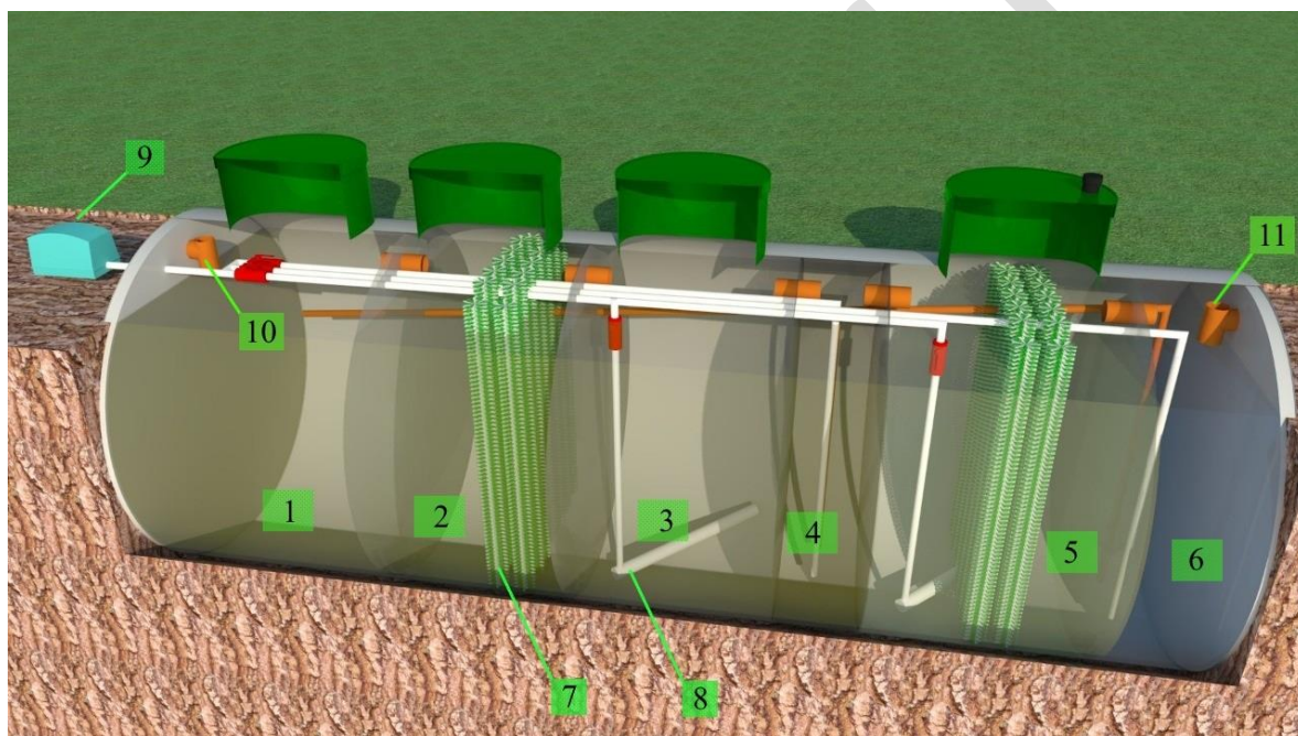
Рис.6.1 Схема ЛОС ЭКО-ЕНОТ «АТЛАНТ»
