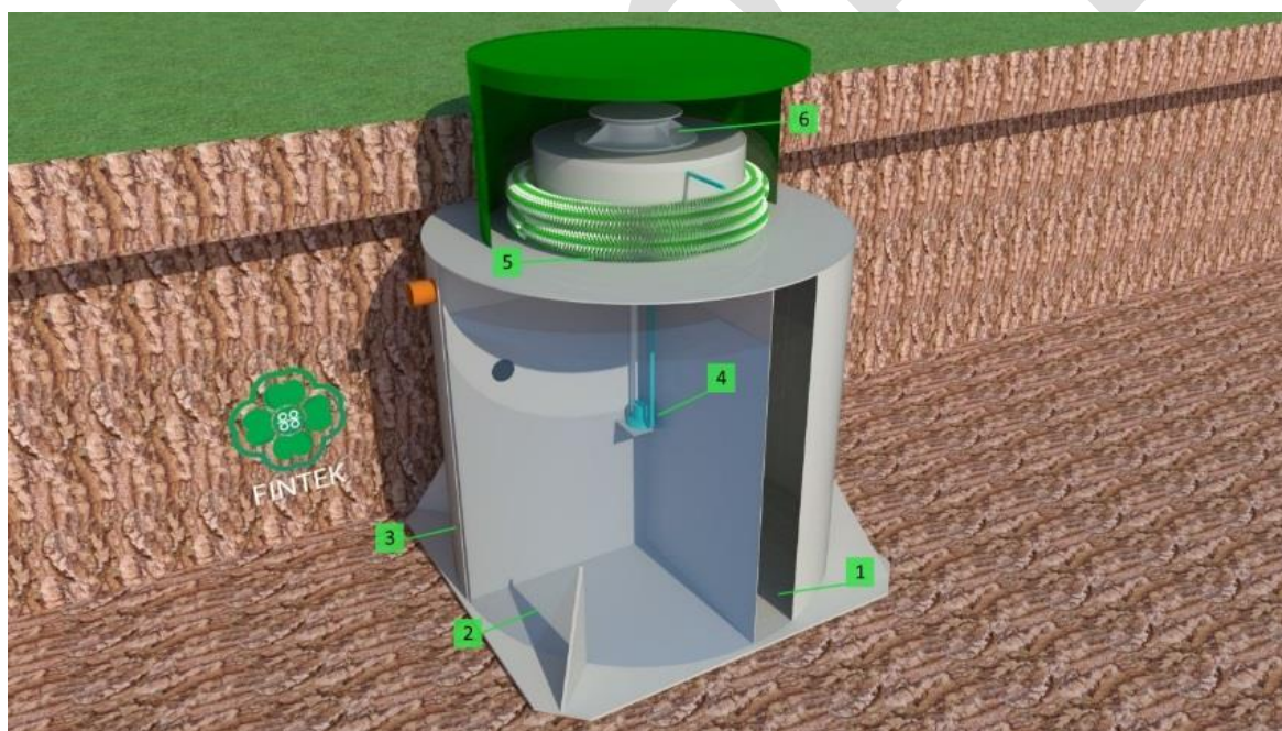
Рис.6.1. Схема ЛОС FINTEK
