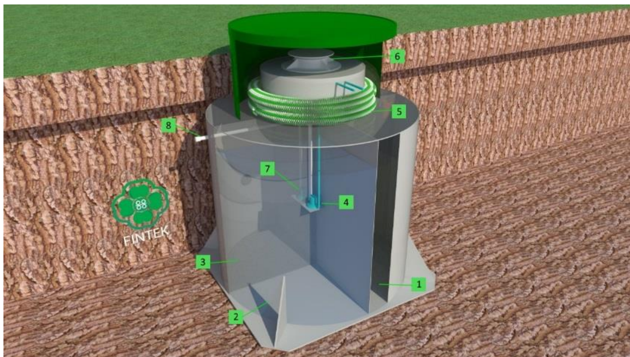
Рис.6.2. Схема ЛОС FINTEK с принудительным сбросом воды
